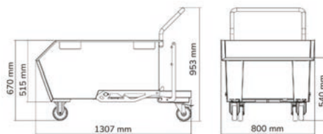
BENNA PORTAROTTAMI RIBALTABILE CAPACITÀ 300 L CON RUOTE PREDISPOSTA PER GRIGLIA E RUBINETTO
