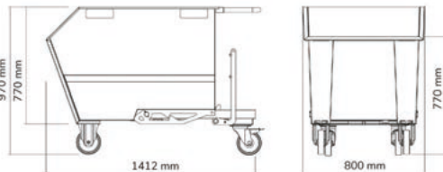
BENNA PORTAROTTAMI RIBALTABILE CAPACITÀ 500 L CON RUOTE PREDISPOSTA PER GRIGLIA E RUBINETTO
